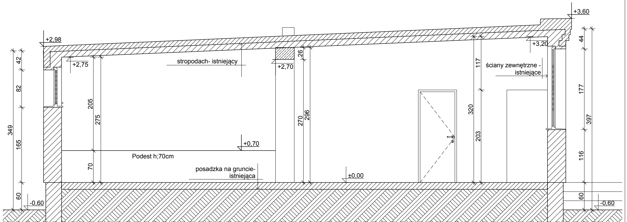
Inwentryzacja- Przekrój A-A
